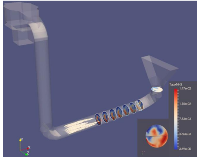
Simulation numérique d'une injection de réactif pour le traitement des fumées dans une gaine de fumées de grandes dimensions
