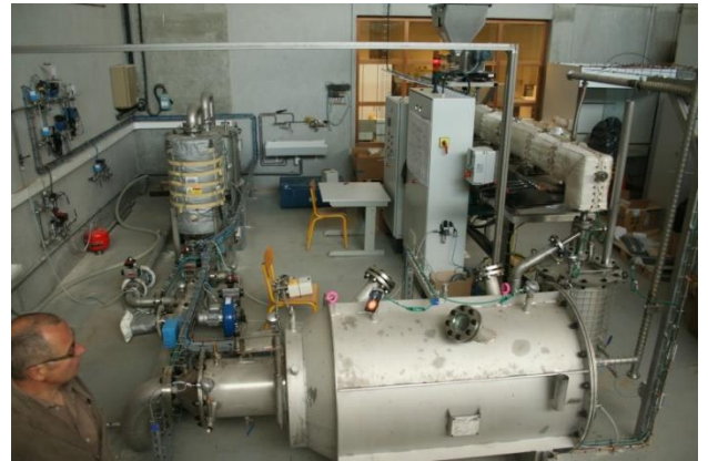
Banc d'essais pour l'étude du traitement des terres contaminées et de la pyrolyse de matières hydrocarbonées mis en place par ATANOR chez PROVADEMSE
