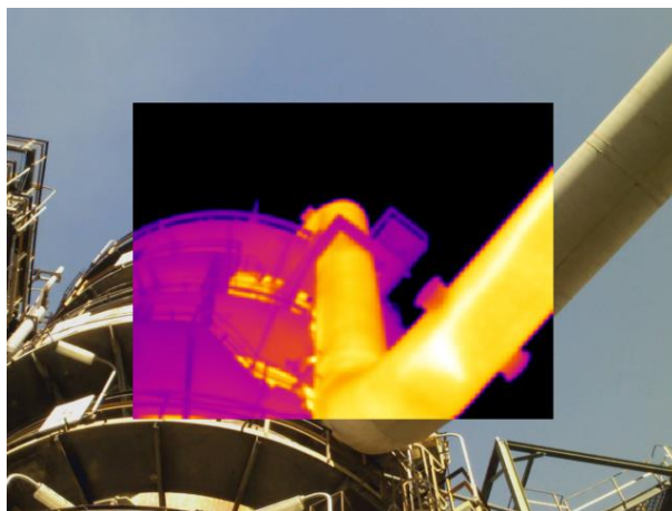
Thermographie d'une conduite de fumées sur unité FCC (craqueur catalytique)
